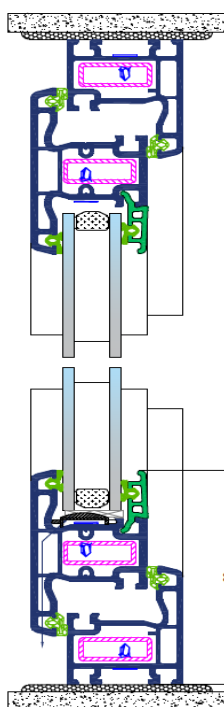
CORTE B - B
